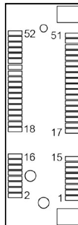
M-PCIE1
