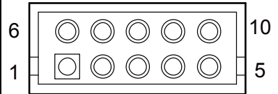
COM3/ COM4 Pin Header
