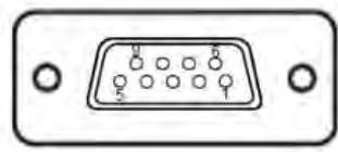
COM3 / COM4
