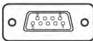
COM1 / COM2
